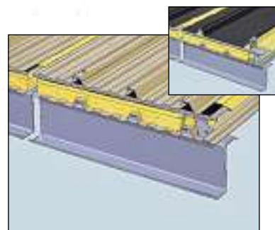
ACOPERIȘUL CU DUBLU STRAT.
