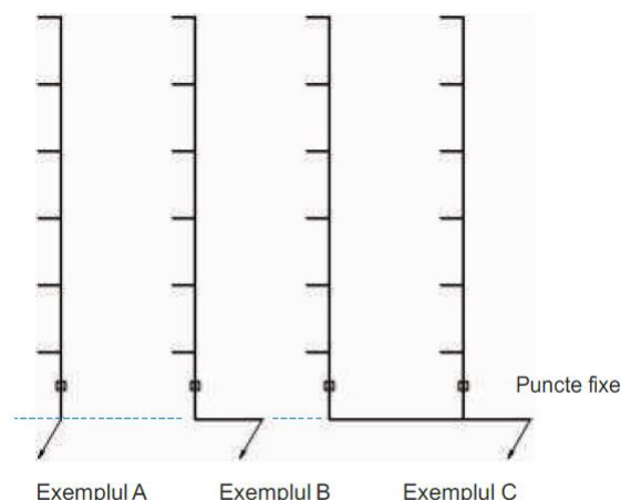
Figura 4.8 Poziția punctelor fixe pentru conductele orizontale
