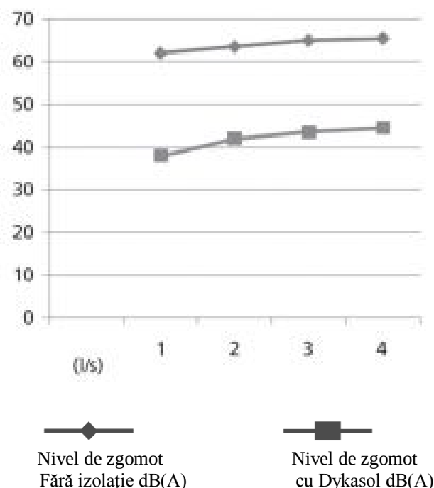
Graficul 2.1 Proprietățile acustice ale izolației Dykasol pentru o coloană de 110mm
