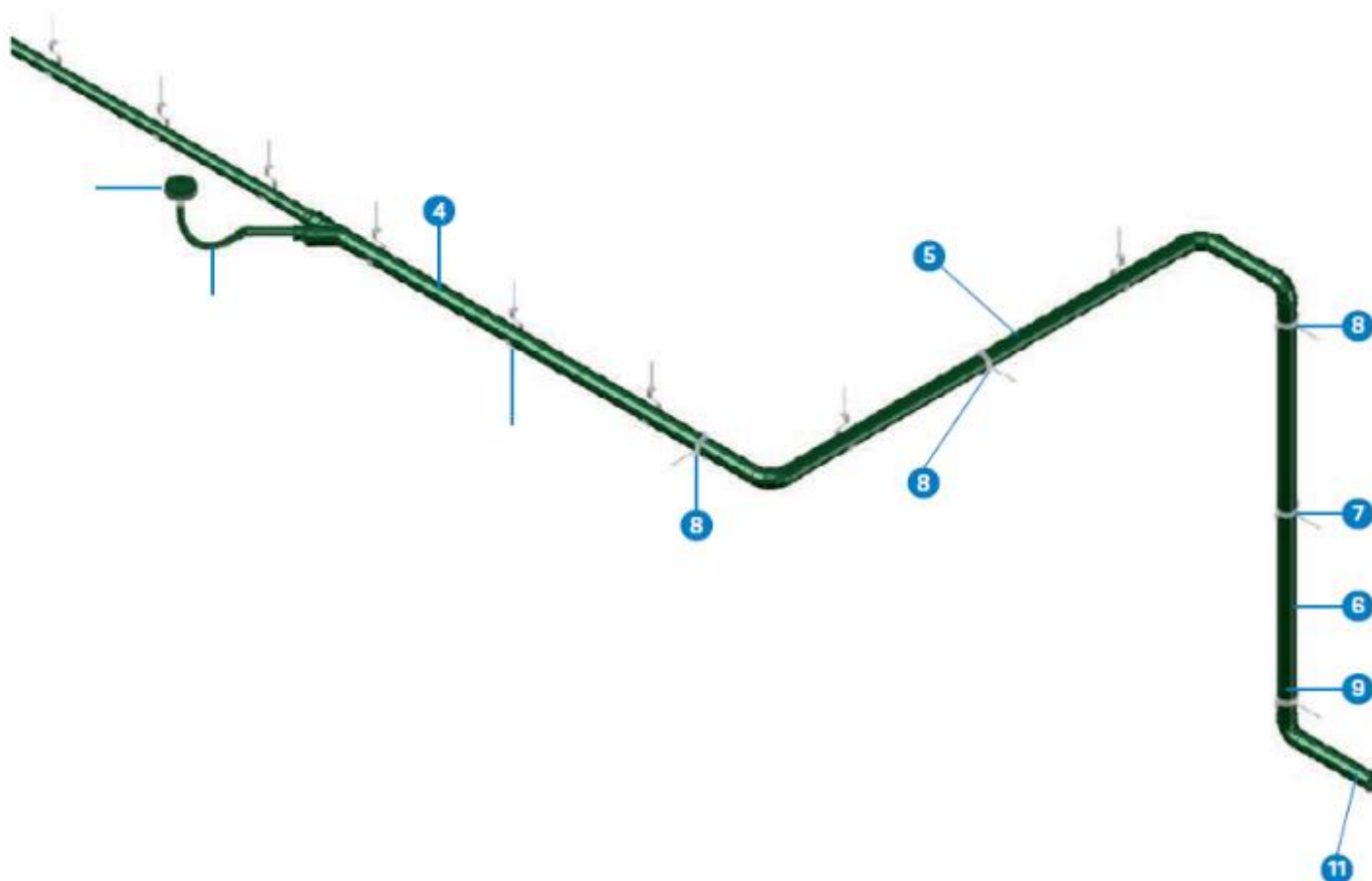
Figura 4.3 Denumirea componentelor din sistemul Vacurain Flex
