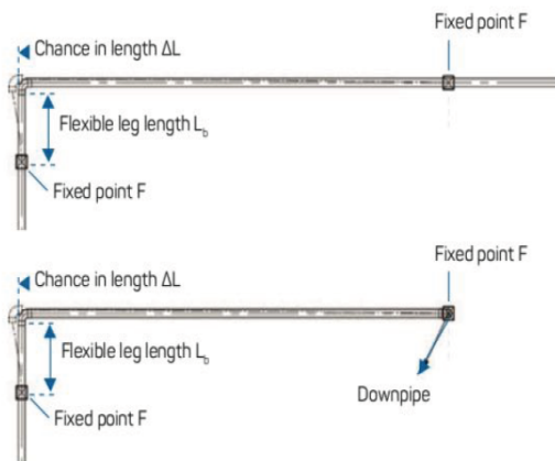
Figura 4.9 Poziția punctelor fixe, poziția secțiunilor de conductă care se deplasează.
