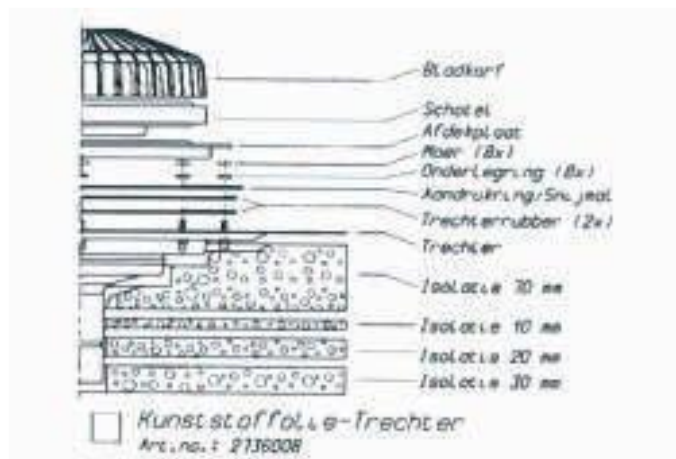
Figura 6.22 Componenta unui ansamblu de receptor
