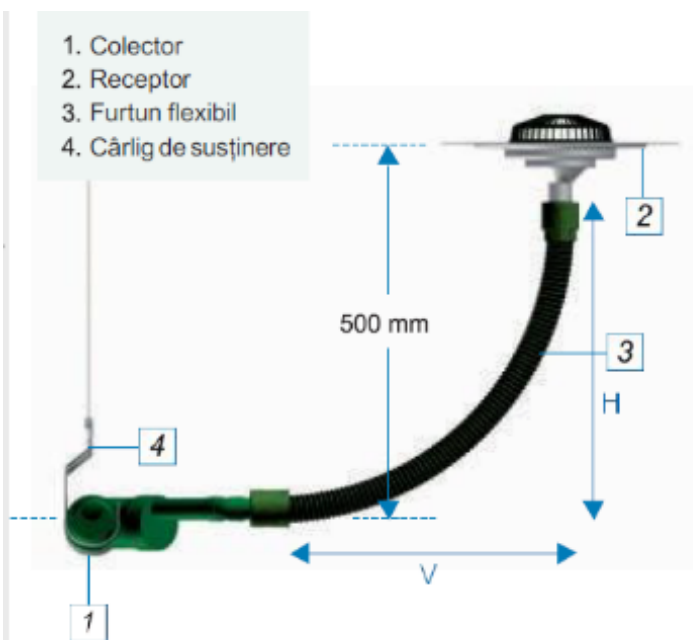
Figura 6.6 Vedere laterală a metodei 1
