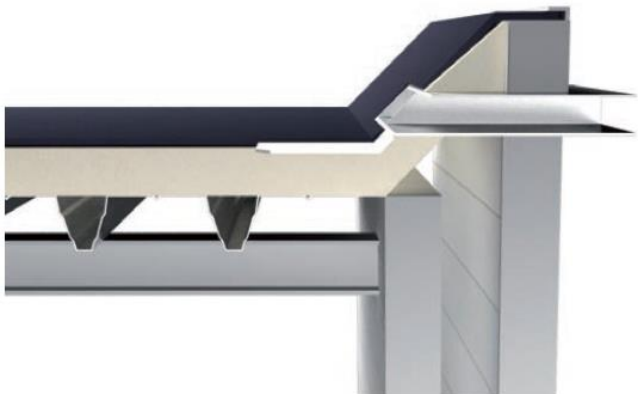
Figura 2.3: Secțiune transversală printr-un element de preaplin
