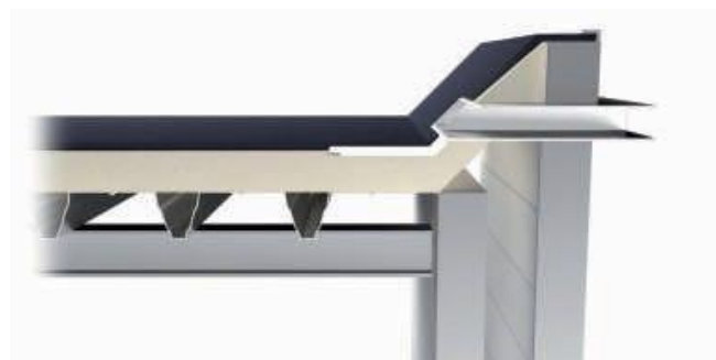
Figura 6.16 Element de preaplin
