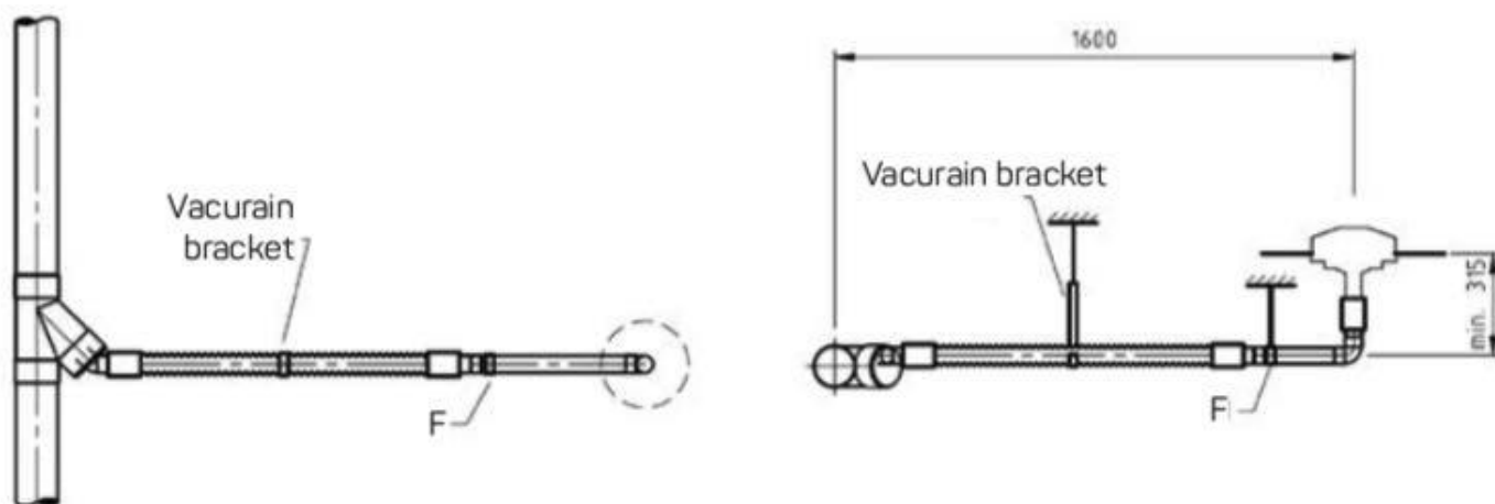
Vedere superioară a conductei și furtunului. receptorului.
