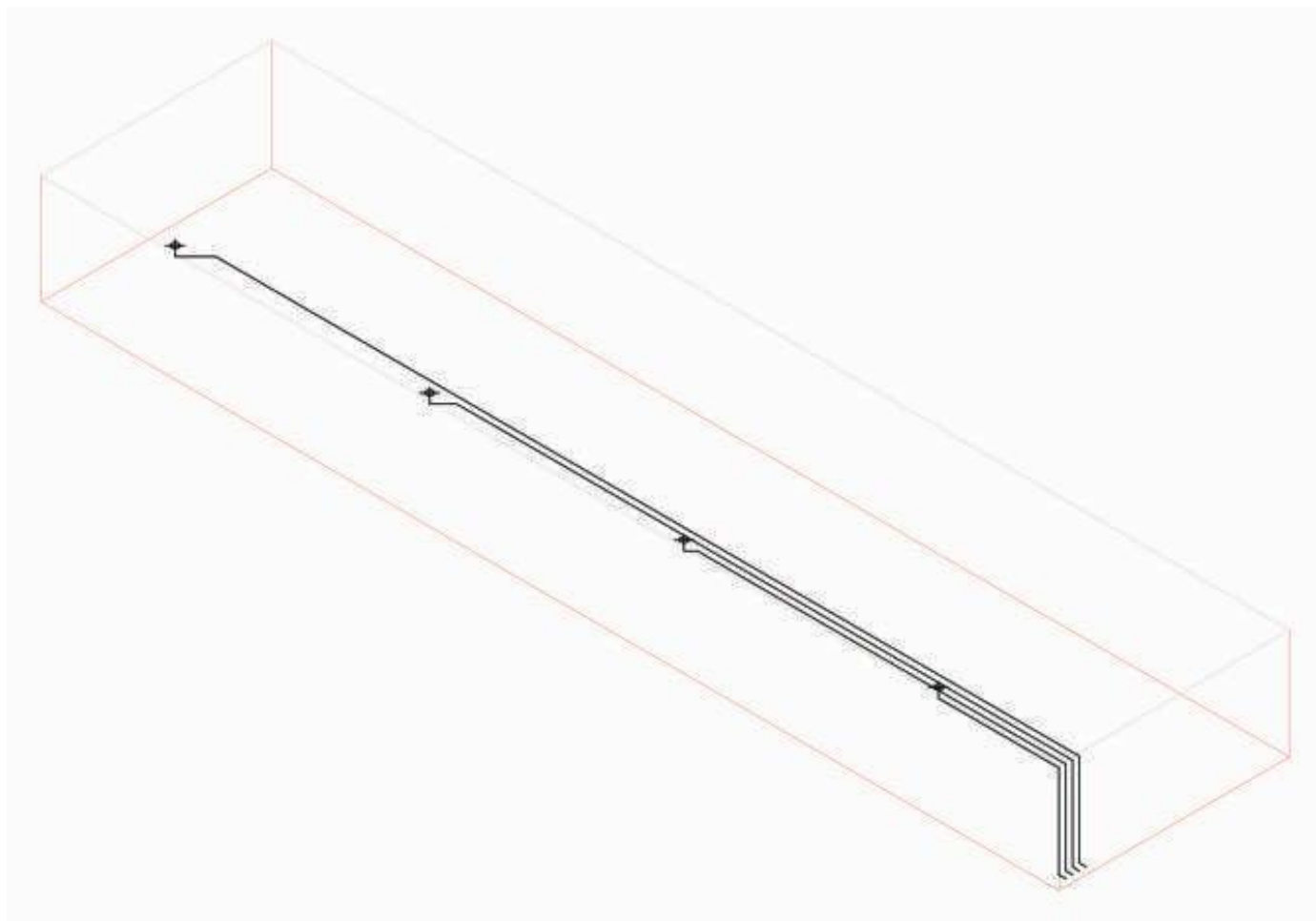
Figura 6.15 Exemplu de un sistem de protecție cu conducte paralele.
